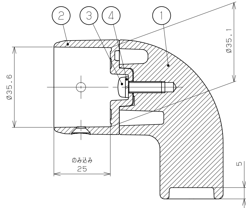
A-A断面図 (S=1/1)
